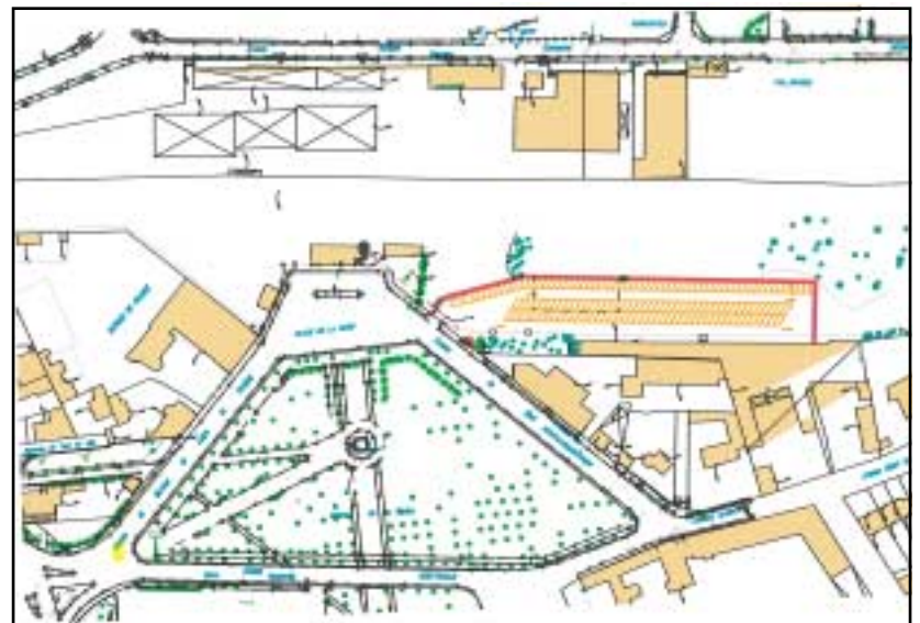
Projet d'implantation du parc de stationnement de 150 places à la gare.
